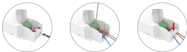
压线安装
